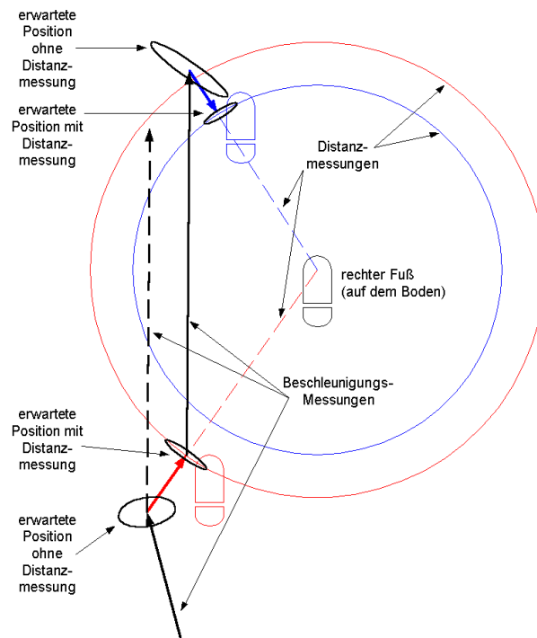
Abbildung 3.4: Foot-to-Foot-System (Bild: nach [Brand and Phillips 2003, S. 116])
