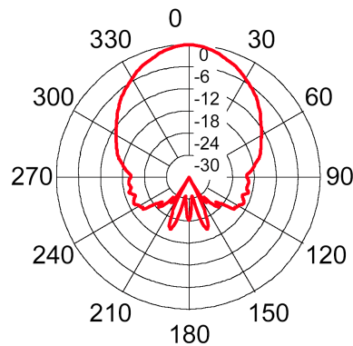
Abbildung 4.16: Öffnungswinkel der Ultraschall-Transmitter und -Receiver (Bild: 12 )
