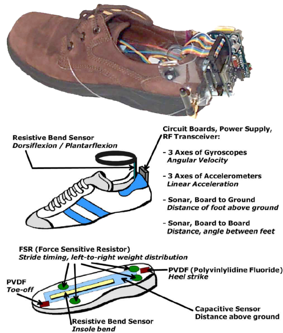
Abbildung 3.1: Instrumented Footwear (Bild: nach [Paradiso et al. 2004, S. 1342])
