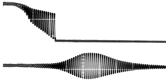
Abbildung 4.15: Oben: gesendetes Signal, unten: empfangenes Signal (siehe auch 4.5.2 Distanzmessungs-Ergebnis)
