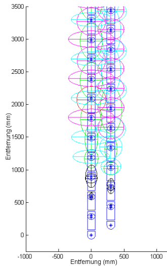
Abbildung 5.8: Fehlerabschätzung mit Geta-Sandals-Werten (Ausschnitt)
