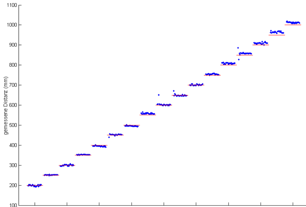
Abbildung 4.20: Gemessene Distanzen von 200 bis 1000 mm bei 60°-Ausrichtung
