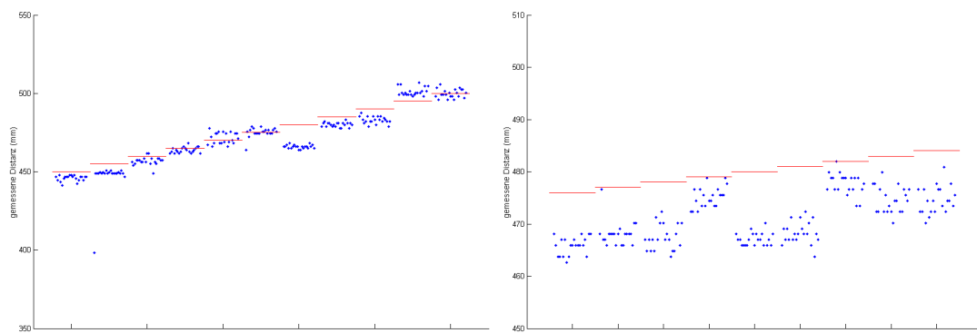
Abbildung 4.21: Gemessene Distanzen bei 60°-Ausrichtung, links: von 450 mm bis 500 mm, rechts: von 476 mm bis 484 mm
