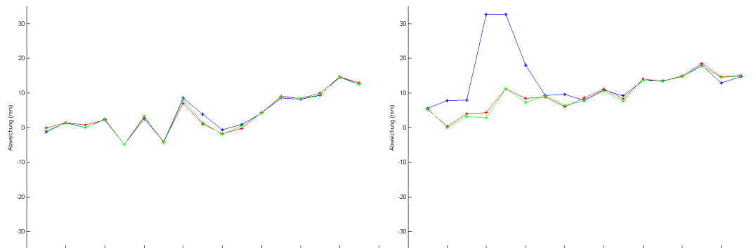
Abbildung 4.26: Ermittelte Abweichung 200 bis 1000 mm, links: harter Untergrund, rechts: weicher Untergrund (blau: Durchschnitt, rot: Median, grün: mittl. Durchschnitt)
