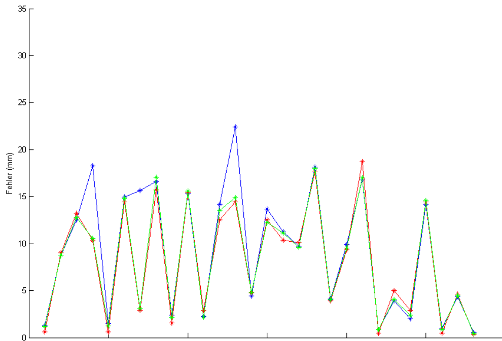
Abbildung 4.25: Ermittelte Fehler bei unterschiedlicher Fußanordnung, wechselnd Distanzmessung zwischen Zehen und Fersen (blau: Durchschnitt, rot: Median, grün: mittl. Durchschnitt)
