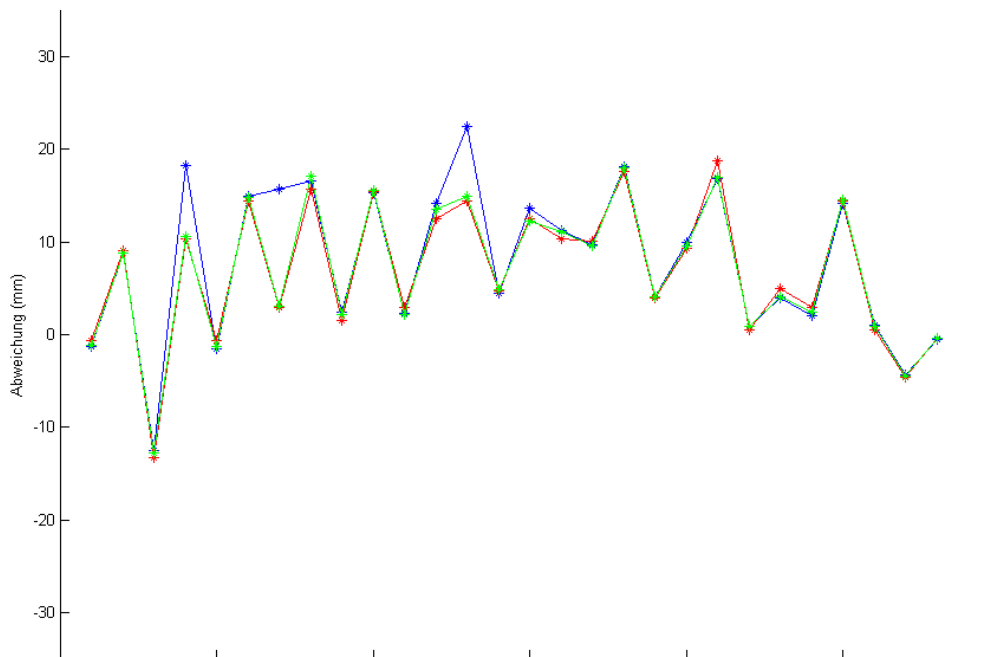
Abbildung 4.27: Ermittelte Abweichung bei unterschiedlicher Fußanordnung, wechselnd Distanzmessung zwischen Zehen und Fersen (blau: Durchschnitt, rot: Median, grün: mittl. Durchschnitt)
