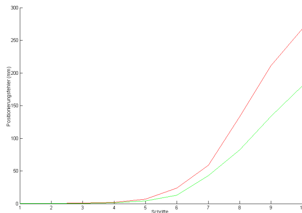
Abbildung 5.1: Positionierungsfehler bei simulierter Messgenauigkeit von 0,01 mm und 10 Schritten (rot: Zehen, grün: Ferse)
