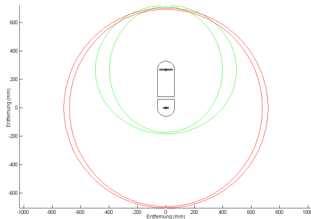
Abbildung 4.10: Ellipsen durch Summierung der Fehler der Ausgangspunkte und der Distanzen
