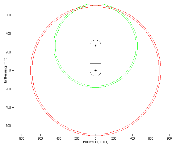
Abbildung 4.7: Kreise der Standardabweichung
