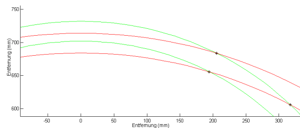
Abbildung 4.12: Es gibt nicht immer Schnittpunkte zwischen allen Ellipsen
