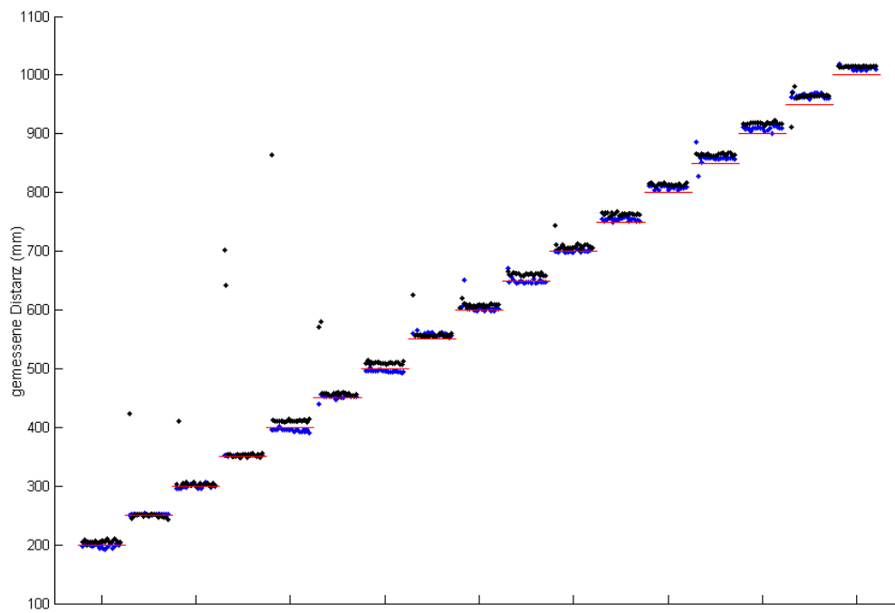
Abbildung 4.23: Gemessene Distanzen (blau: harter, schwarz: weicher Untergrund)
